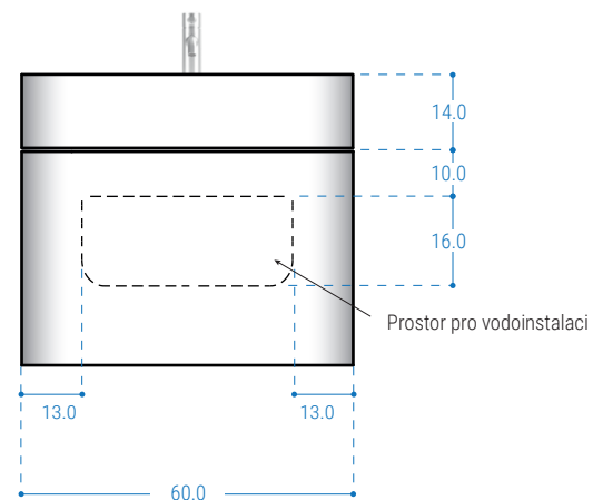
Pohled zepředu
